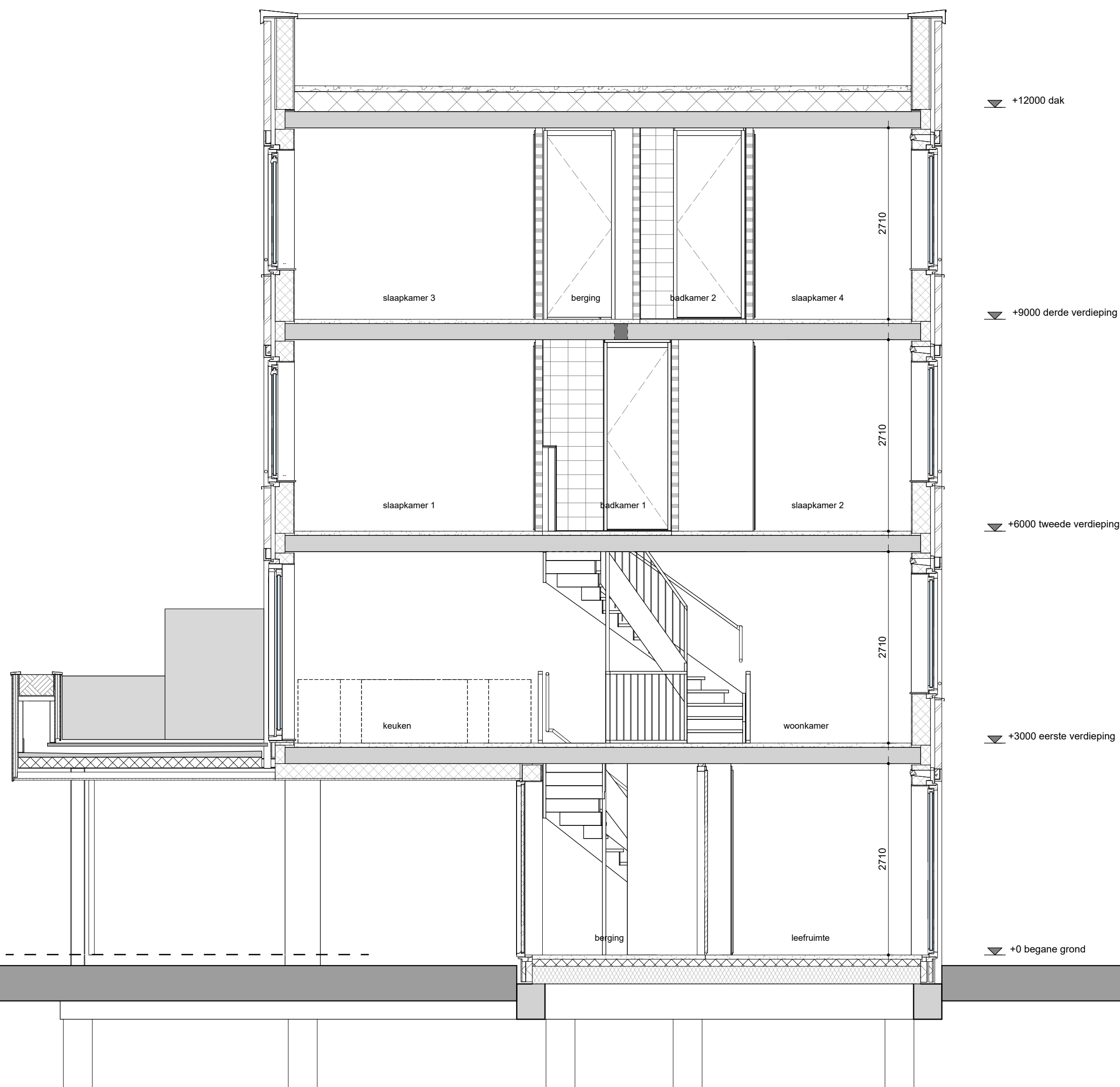
Doorsnede woningtypes G
